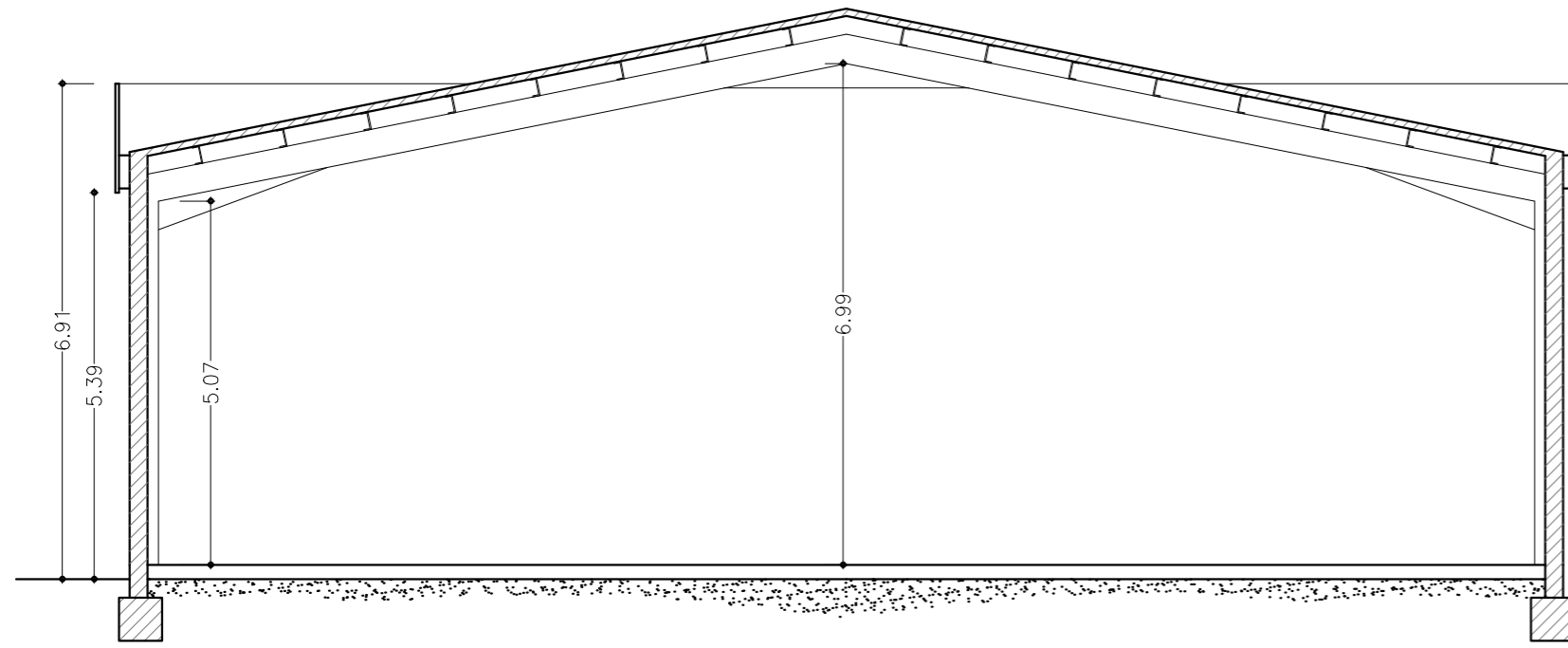
SECCIÓN TRANSVERSAL
